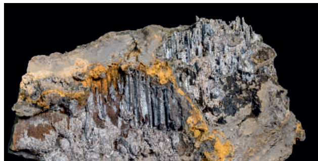
Manganeso oxidoak (rancieita batez ere) eta goethita/Óxidos de Manganeso (principalmente rancieita) y goethita
